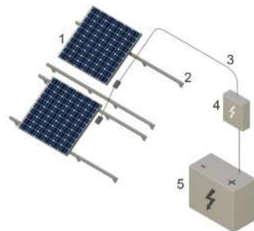
Slika 2: Fotonapetostna naprava
